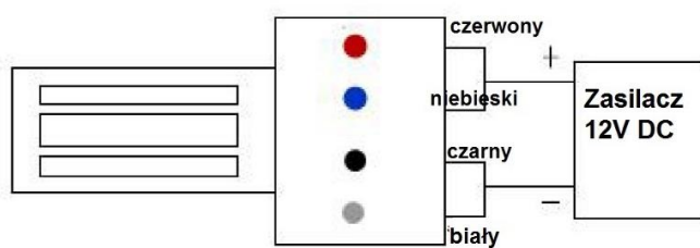
Zasilanie 12V DC
