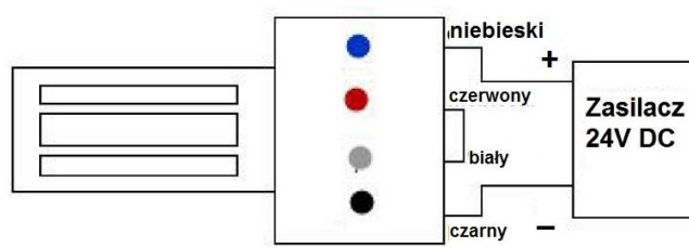
Zasilanie 24V DC
